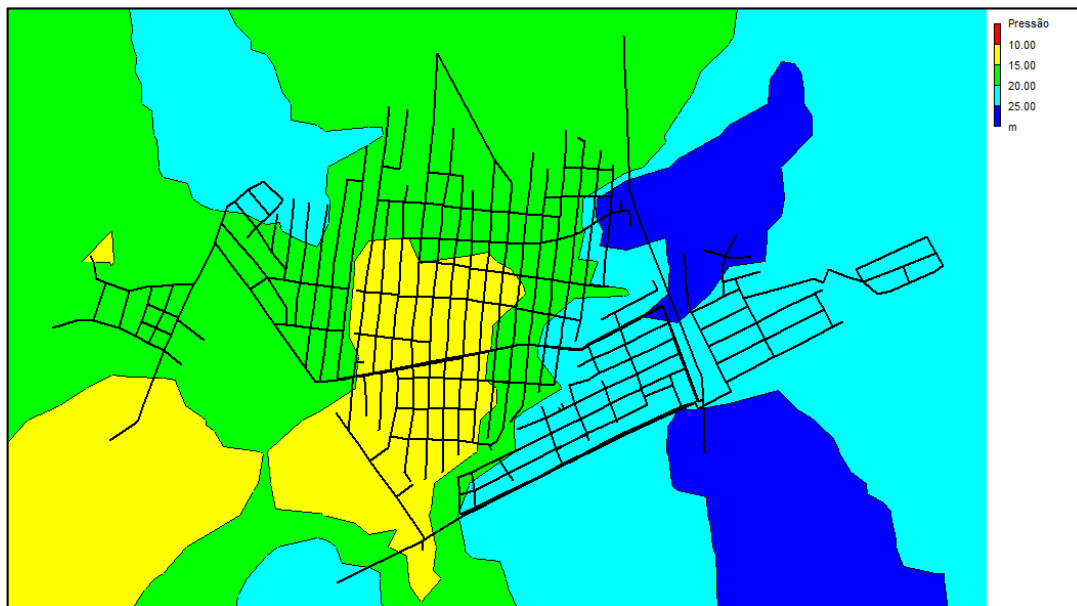
Figura 18: Gráfico de Isolinhas de Pressão – DMC Conjunto Metropolitano
