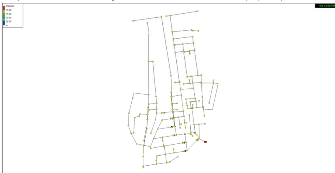
Figura 23: Rede de distribuição modelada no software EPANET proposta para o DMC São Miguel
