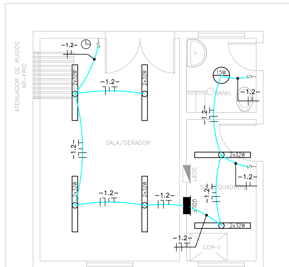
1 PLANTA BAIXA - ILUMINAÇÃO INTERNA ESCALA 1/50
