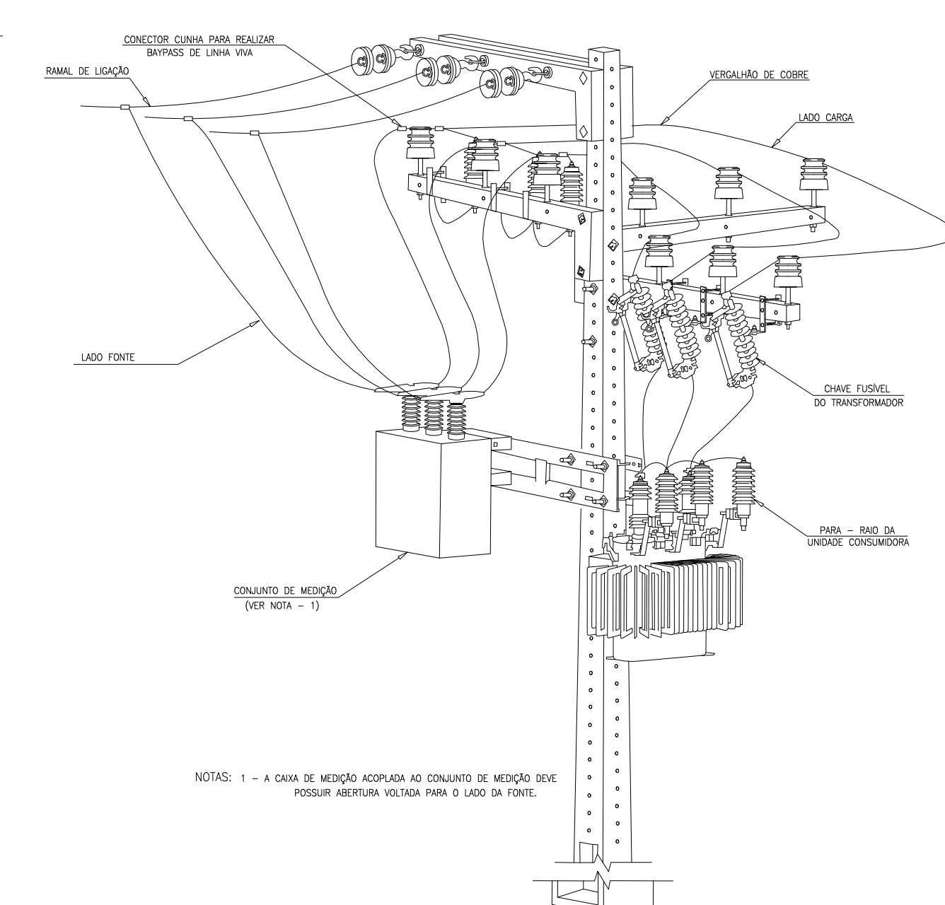
4 VISTA ISOMÉTRICA ESCALA 5/8"
