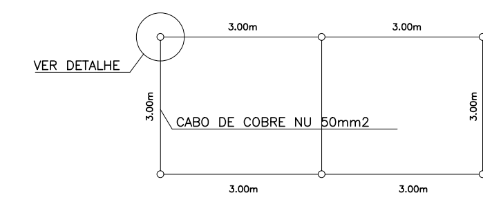
1 ATERRAMENTO ESCALA 1/75
