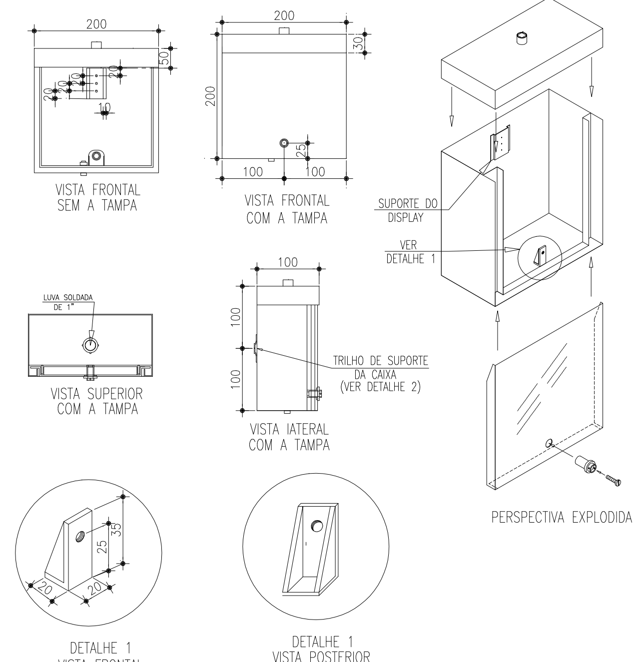
5 DETALHE DO DISPLAY ESCALA 5/8"
