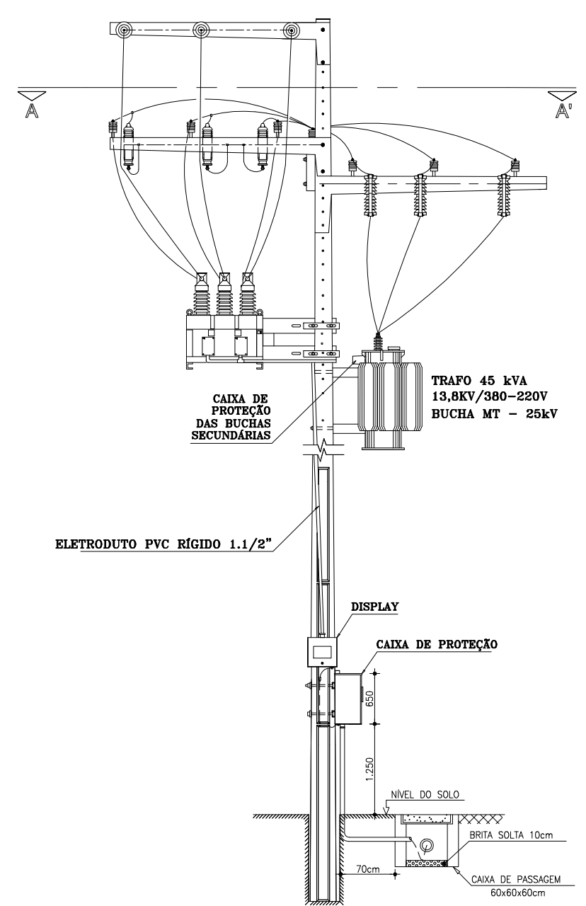
2 VISTA LATERAL ESCALA 5/8"
