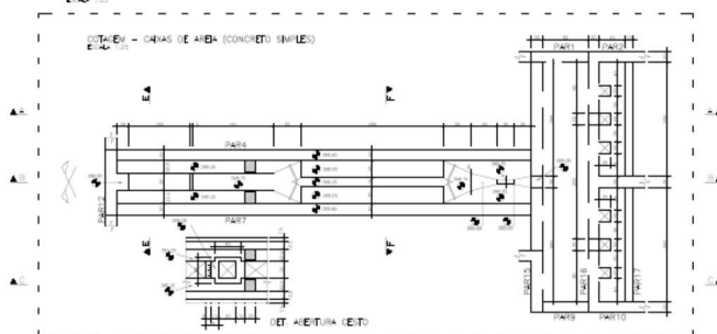
DETALHES – CAIXA DE AREIA / LEITO DE SECAGEM / TANQUE DE SOLUÇÃO DE CAL
