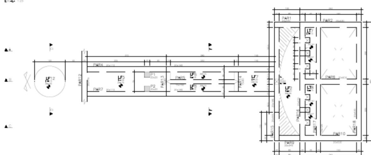
DETALHES – CAIXA DE AREIA / LEITO DE SECAGEM / TANQUE DE SOLUÇÃO DE CAL
