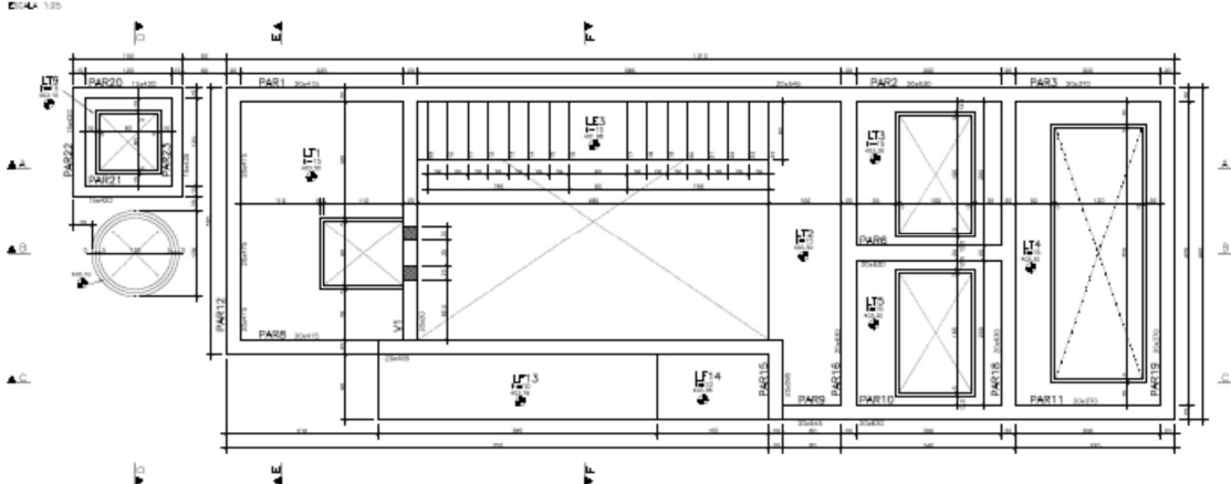
Figura 5: Fôrma da tampa – EEE / SB.9 – plano 1-1 (folha 07/07).
