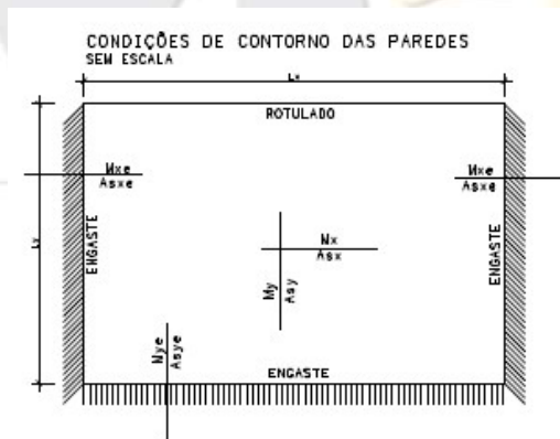
Figura 3: Condições de contorno das paredes.
