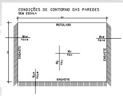
Figura 3: Condições de contorno das paredes.
