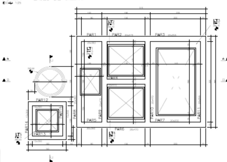
Figura 5: Fôrma da tampa – EEE / SB.5.1 (folha 02/02).
