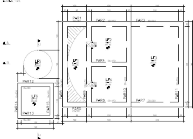
Figura 4: Fôrma dos Fundos – EEE / SB.5.1 (folha 01/02).
