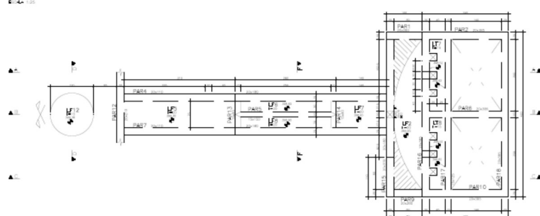
DETALHES – CAIXA DE AREIA / LEITO DE SECAGEM / TANQUE DE SOLUÇÃO DE CAL
