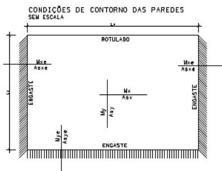
Figura 3: Condições de contorno das paredes.
