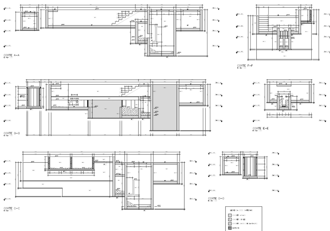
Figura 1: Cortes esquemáticos da EEE / SB.4.
