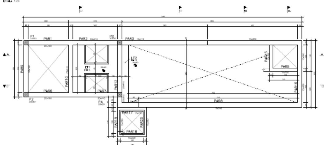
Figura 5: Fôrma da térreo/tampa – EEE / SB.3.2 (folha 06/06).
