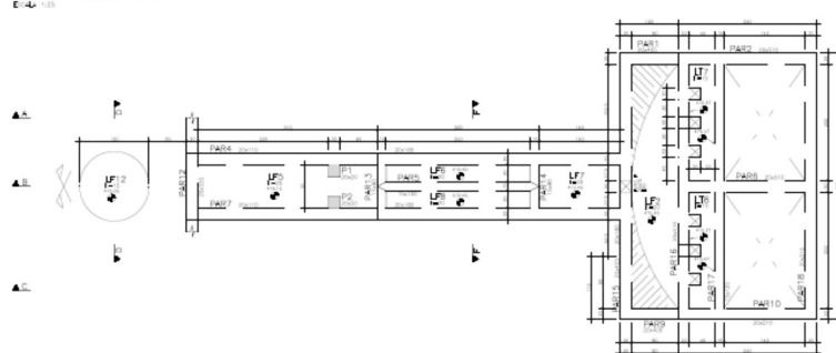
DETALHES – CAIXA DE AREIA / LEITO DE SECAGEM / TANQUE DE SOLUÇÃO DE CAL E=4/1,00
