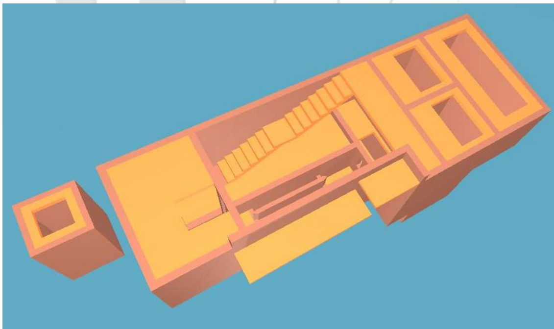
Figura 2: Modelo 3D da EEE / SB.1.
