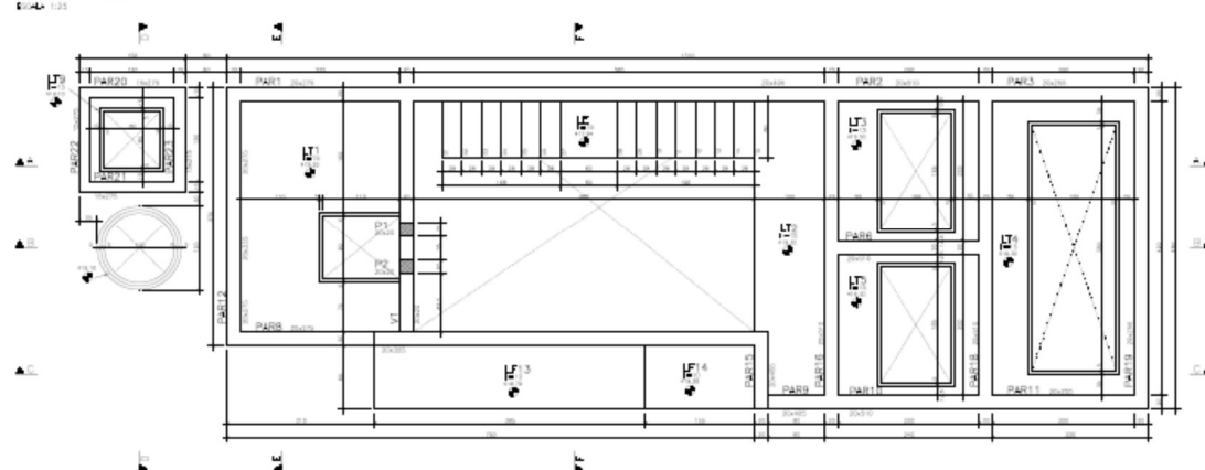
Figura 5: Fôrma da tampa – EEE / SB.1 – plano 1-1 (folha 06/06).
