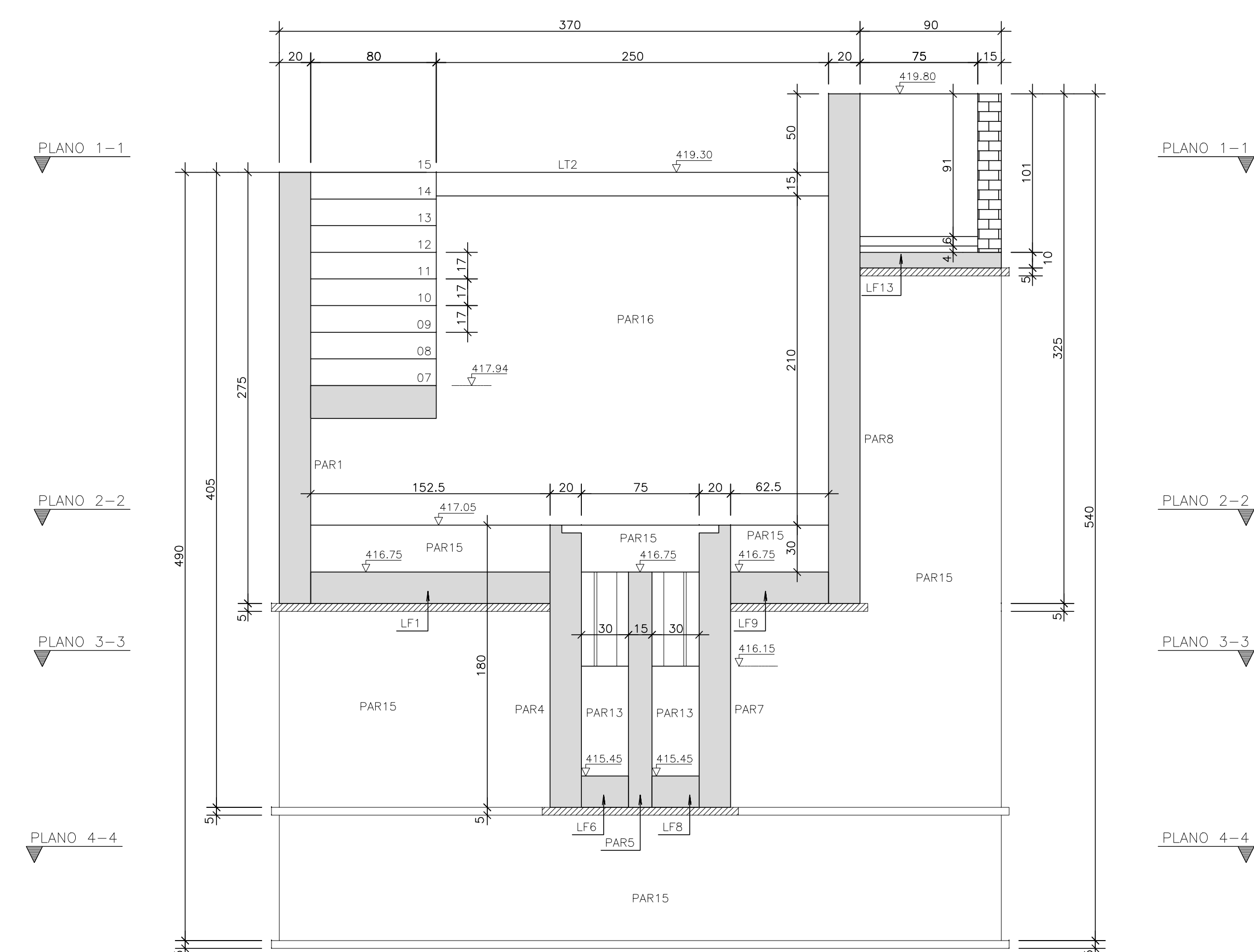
CORTE F-F ESCALA 1:25
