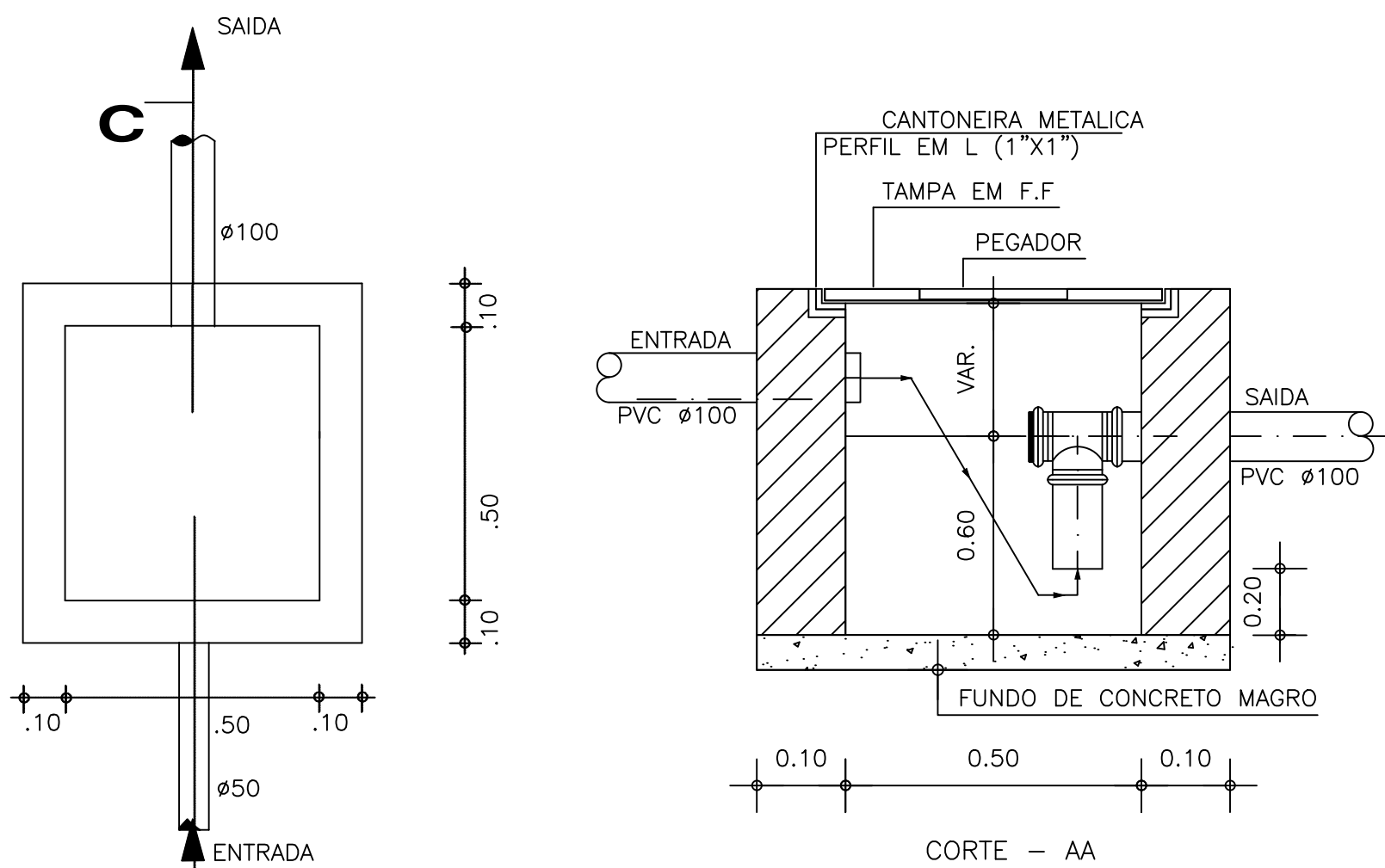
DETALHE CX. DE GORDURA E/OU CX. DE SABÃO SEM ESCALA
