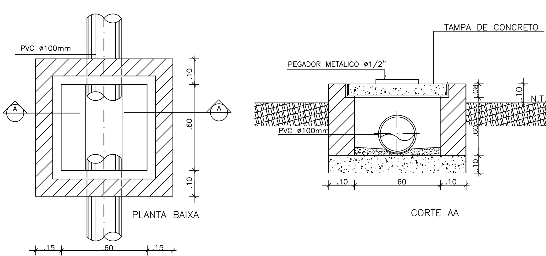
DETALHE CAIXA DE INSPEÇÃO SEM ESCALA
