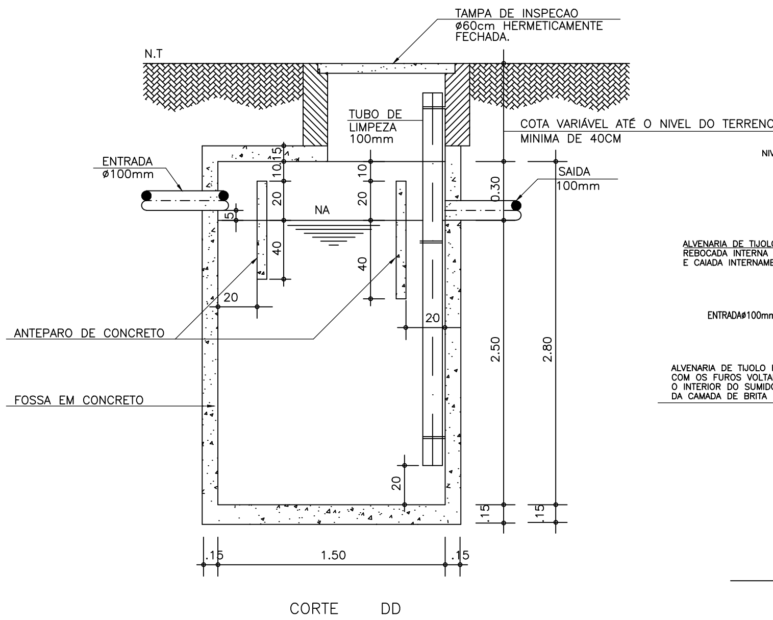
DETALHE FOSSA SEM ESCALA
