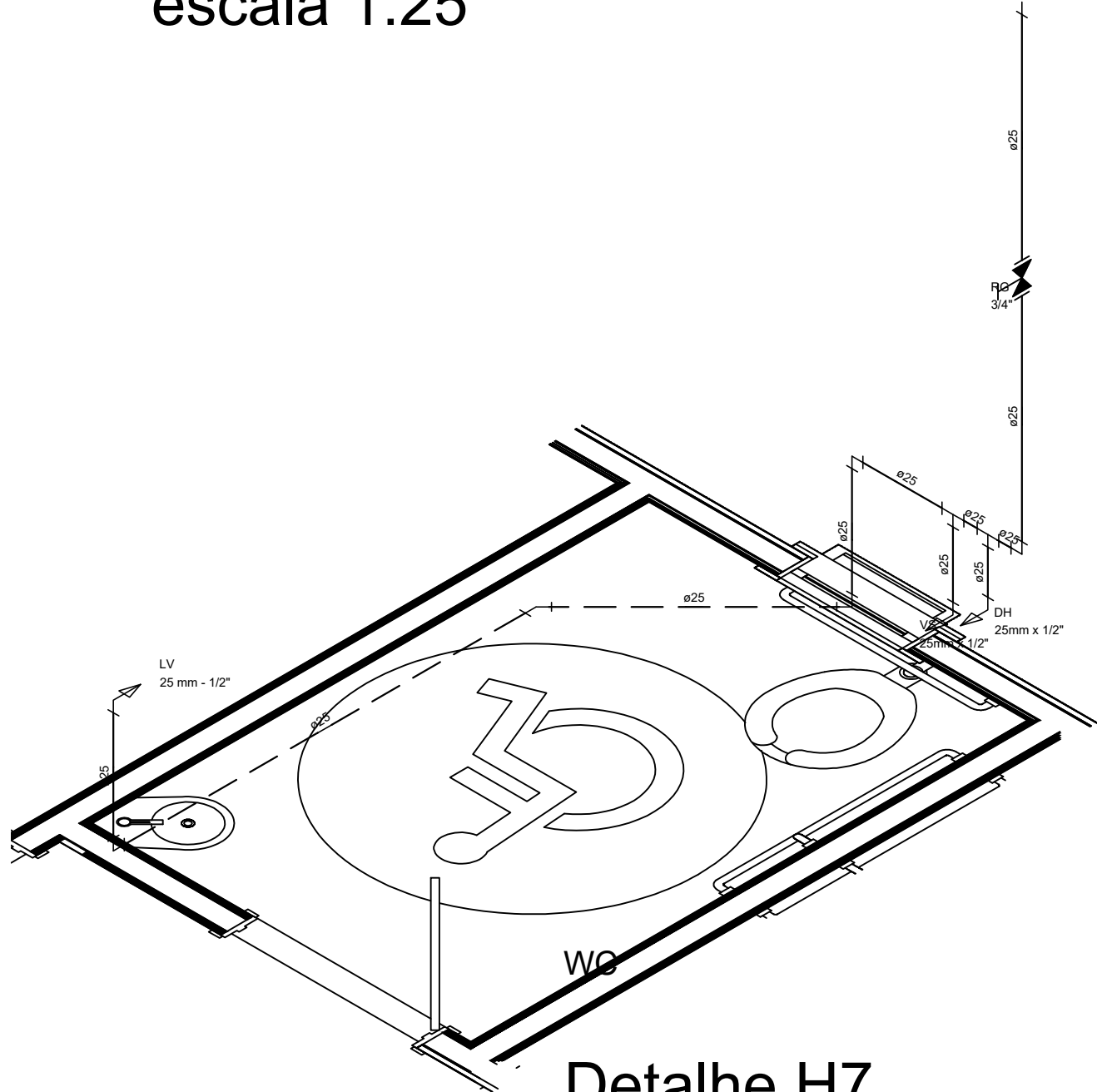
Detalhe H7 escala 1:25
