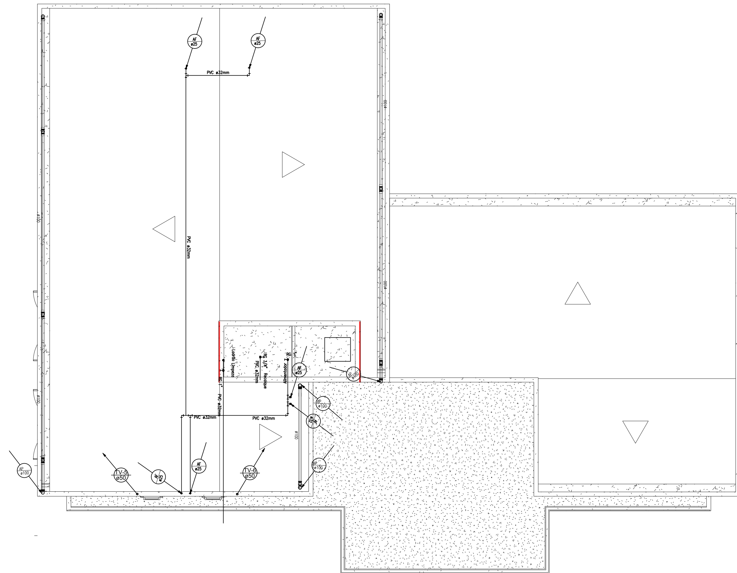
02 | Planta Baixa Coberta - Hidrossanitário Esc. 1/75
