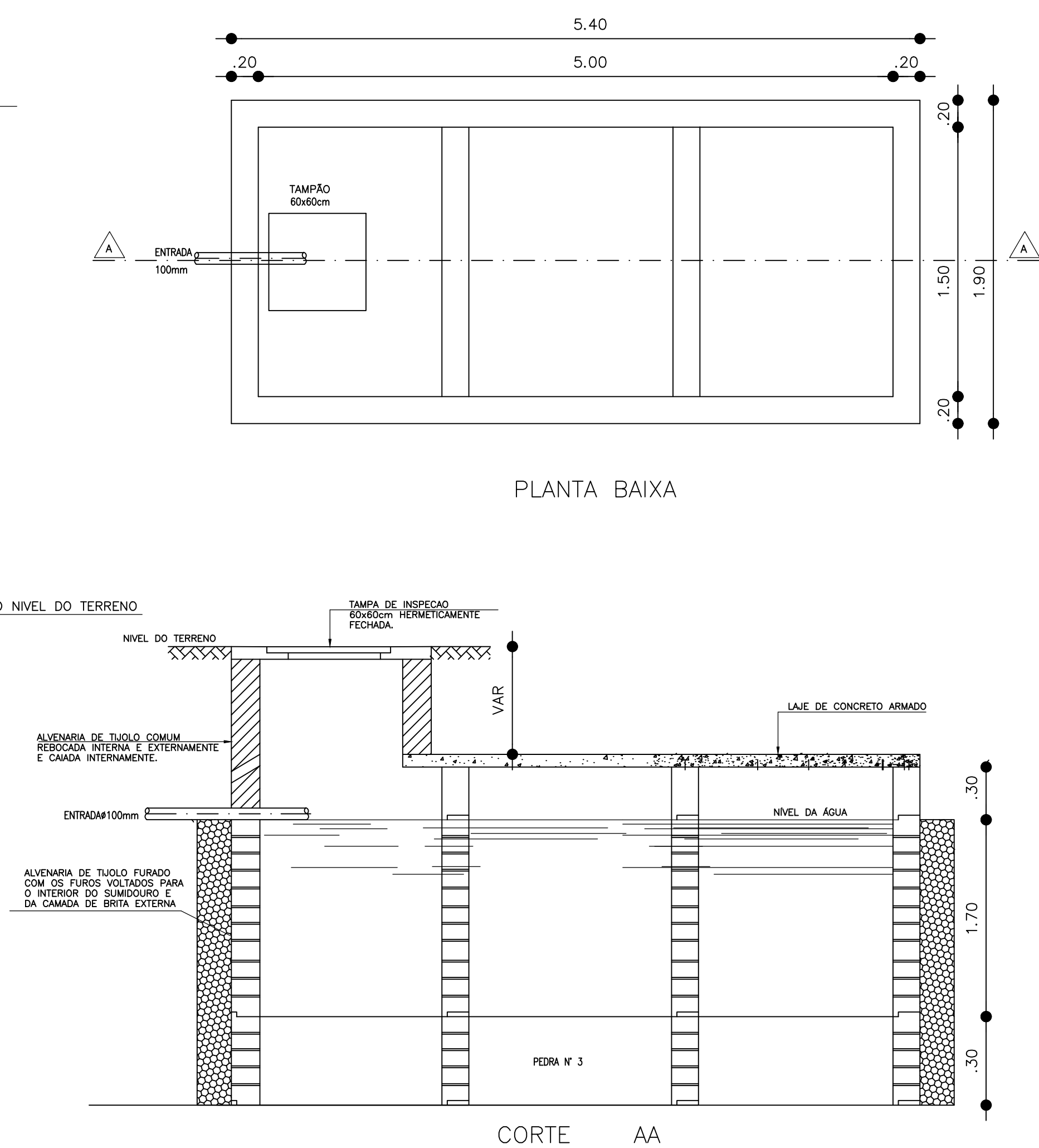
DETALHE DO SUMIDOURO SEM ESCALA
