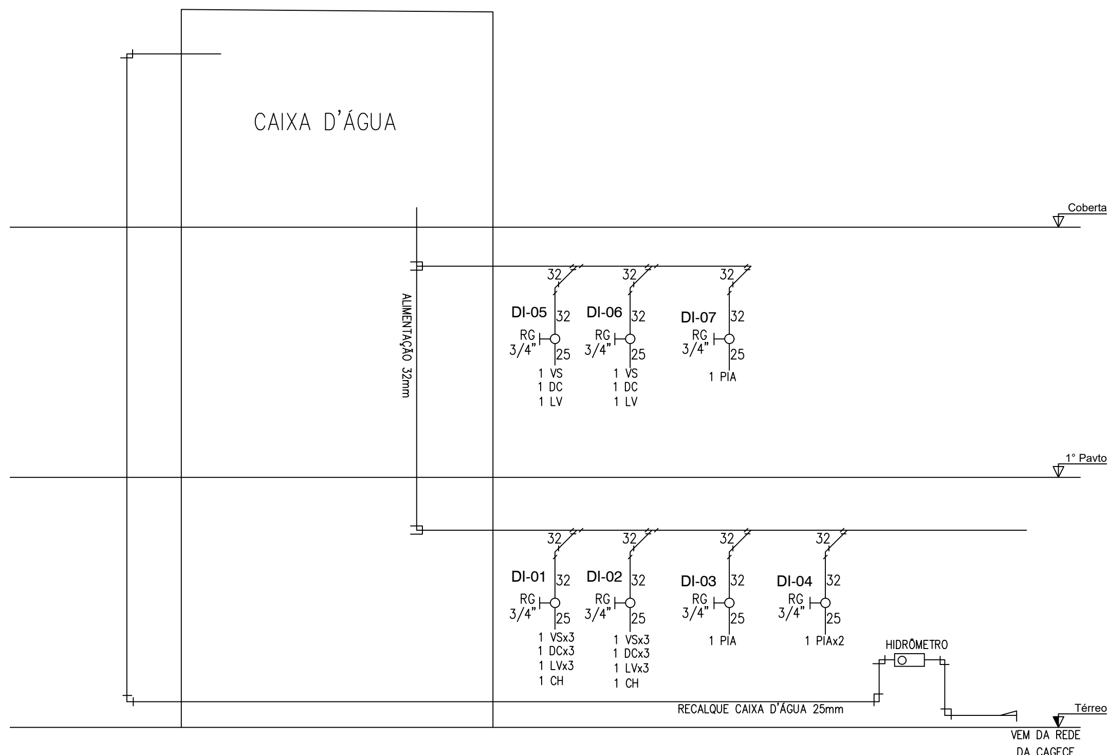
04 | Esquema Vertical - Hidraulica Esc. s/esc
