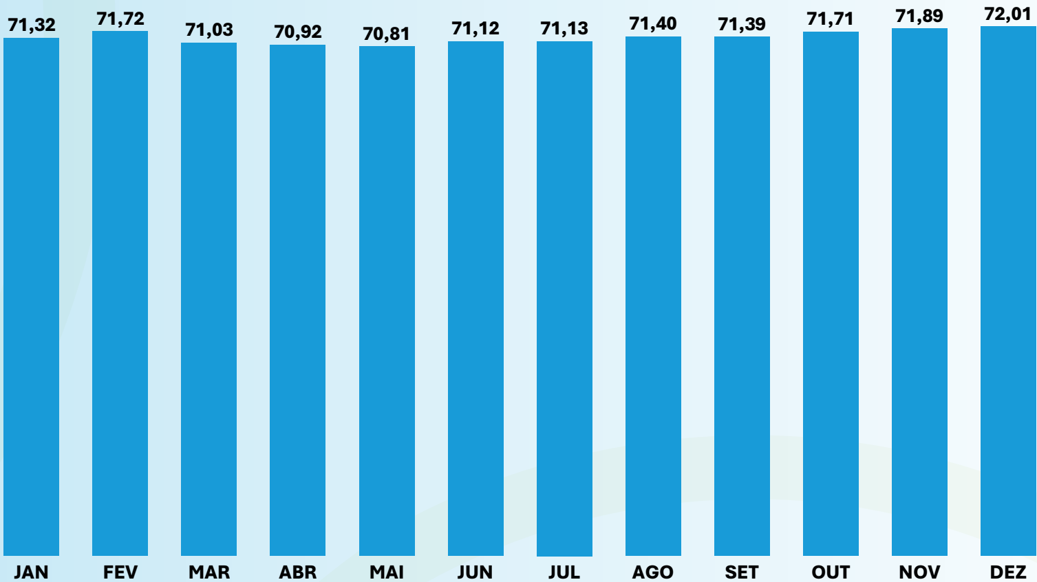
Figura 5: Índice de Utilização da Rede de Água em 2024
