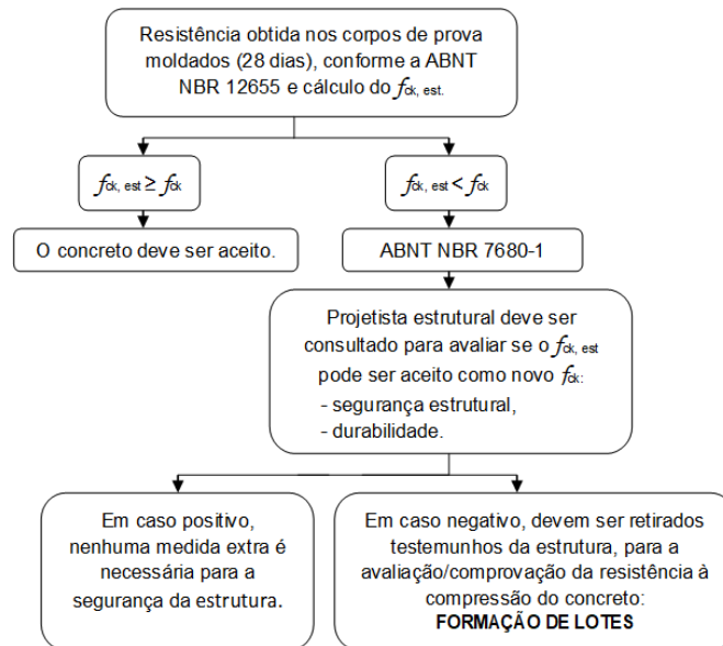
Figura 2 - Análise dos resultados pelo projetista estrutural
